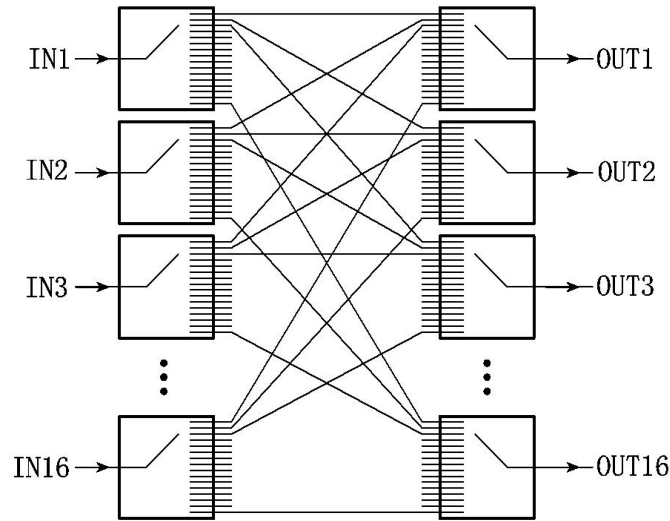
16×16 光开关内部光路示意图
