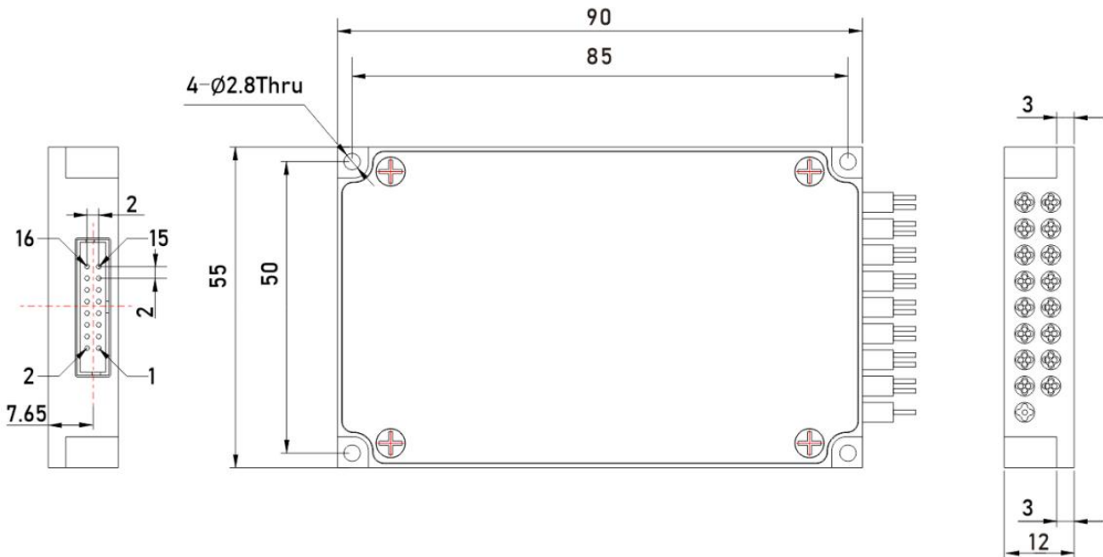
图 2 外型尺寸图 (M3: 90×55×12mm)
