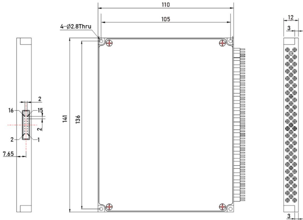
图4 外型尺寸图 (M5: 110×141×12mm)
