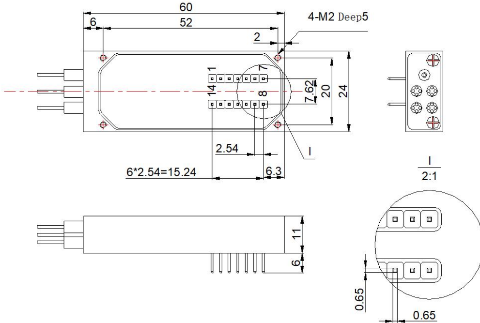
图 1 外型尺寸图 (M2: 60×24×11mm)
