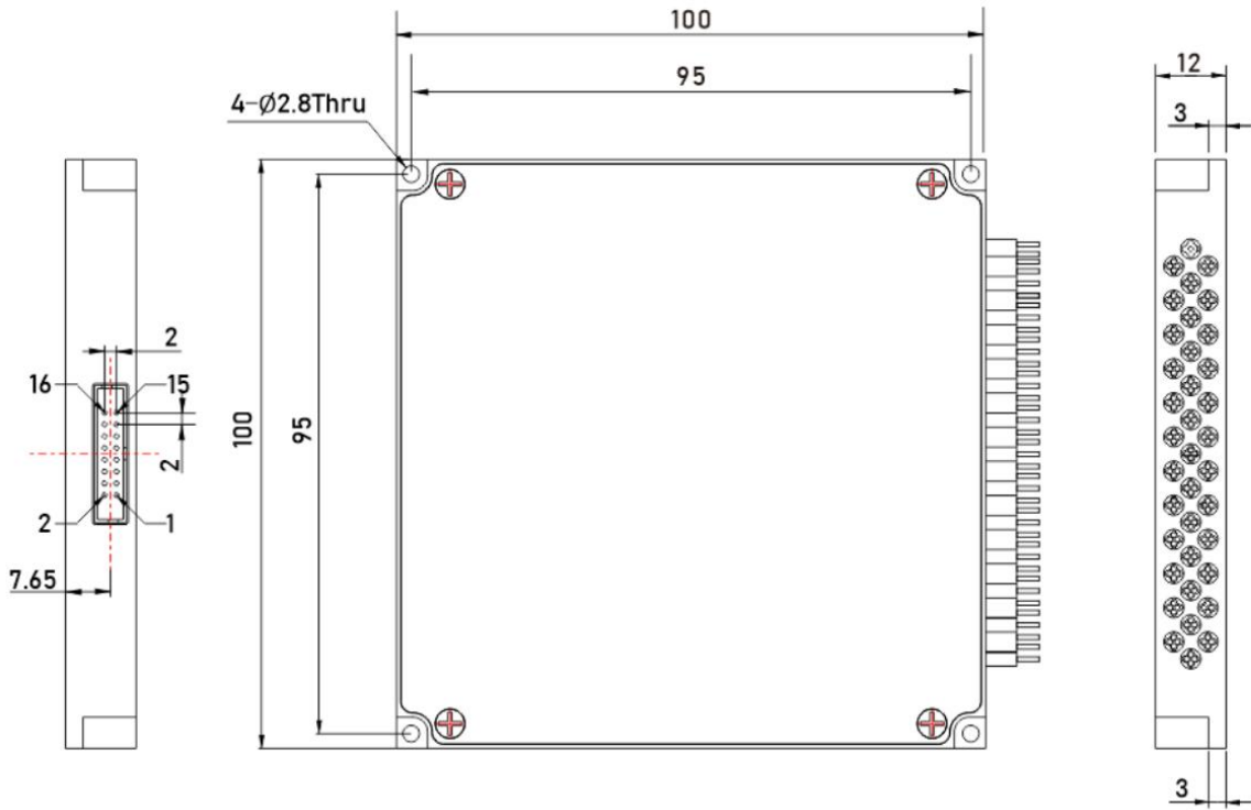
图3 外型尺寸图 (M4: 100×100×12mm)
