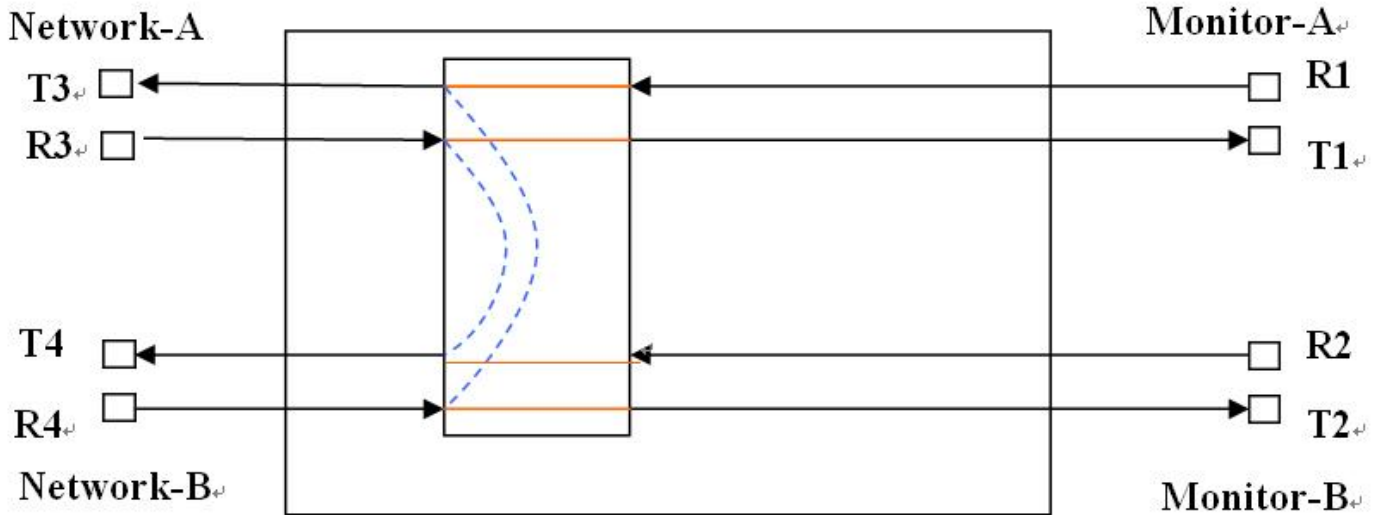
光路示意图
