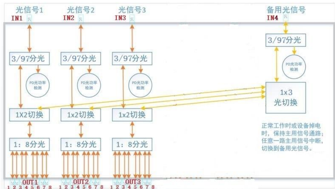
4×3 光开关内部光路示意图
